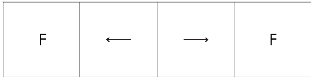
Τετράφυλλο επάλληλο - φιλιτό σε διπλό οδηγό (με δύο σταθερά φύλλα)
