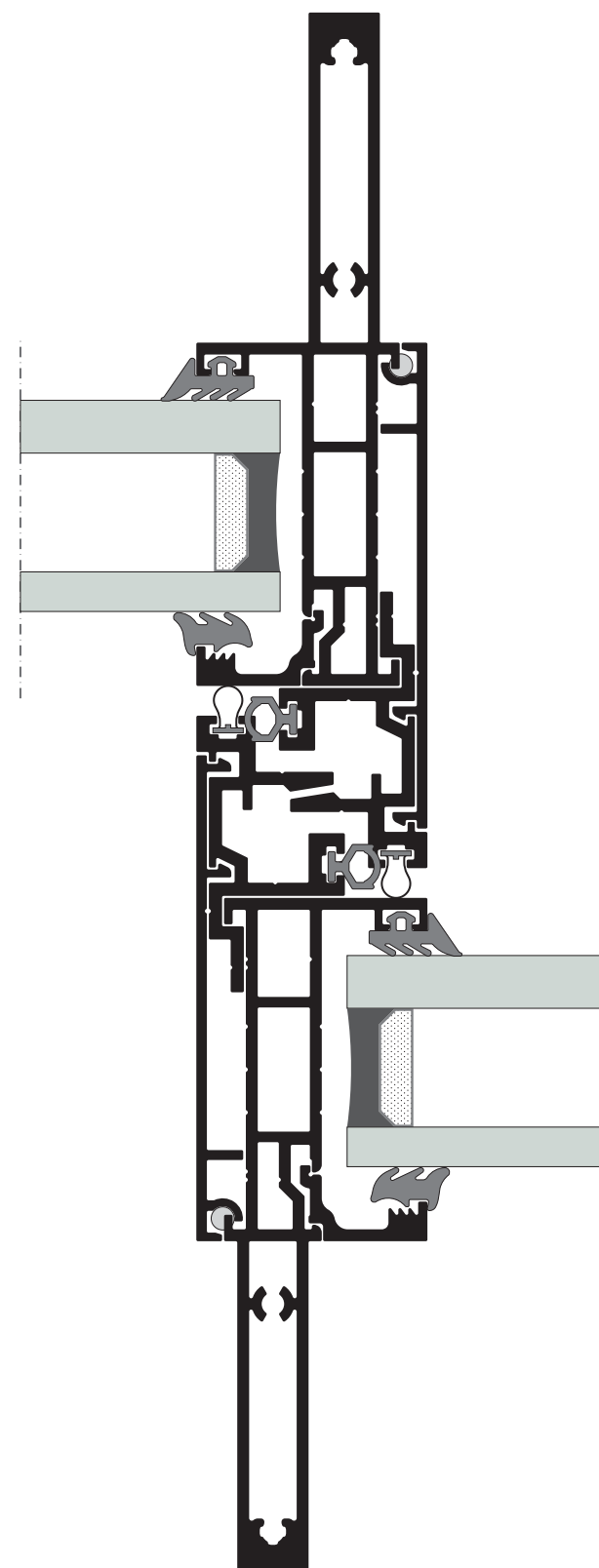
Έκδοση με εσωτερική και εξωτερική ενίσχυση
