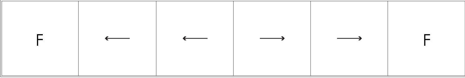
Εξάφυλλο επάλληλο - φιλιτό σε τριπλό οδηγό (με δύο σταθερά φύλλα)
