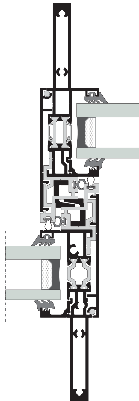
Έκδοση με εσωτερική και εξωτερική ενίσχυση
