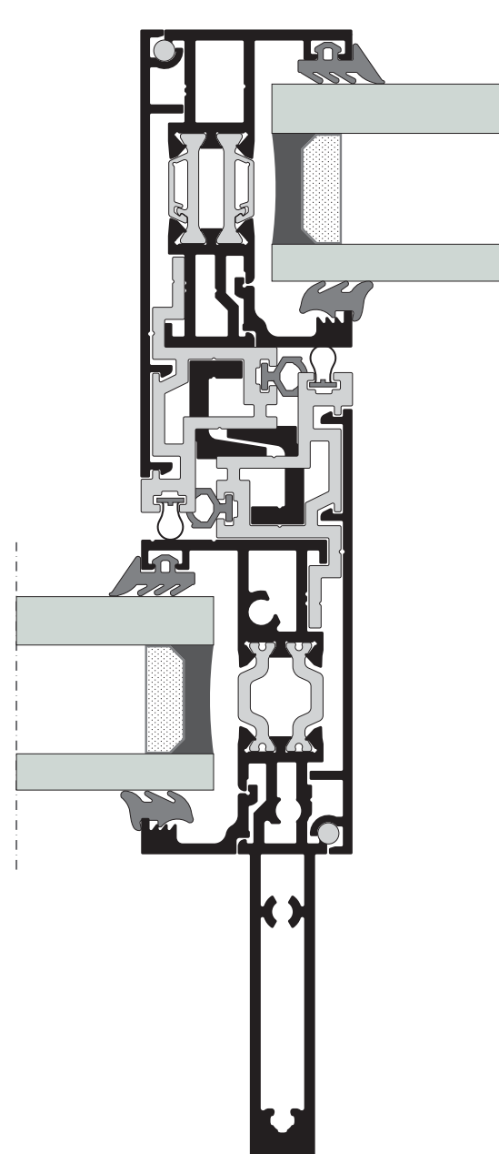
Έκδοση με εσωτερική ενίσχυση
