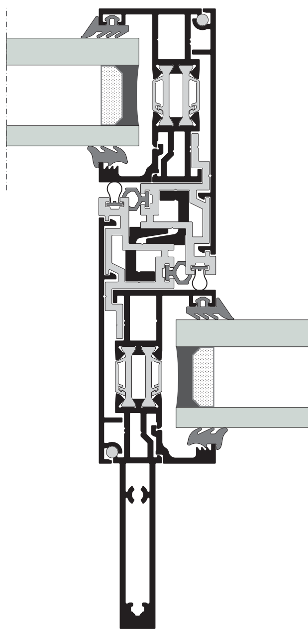
Έκδοση με εσωτερική ενίσχυση
